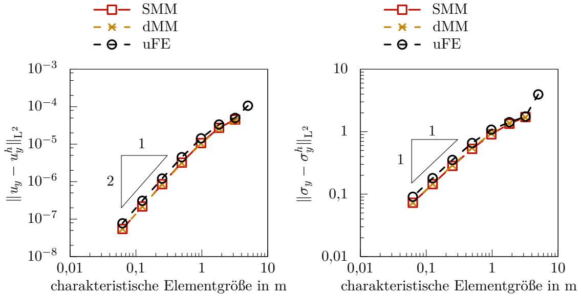
Abbildung 6.2: Einführungsbeispiel: Absoluter Fehler von u_y (links) und \sigma_y (rechts) in der L^2 -Norm in Abhängigkeit der Netzfeinheit.
