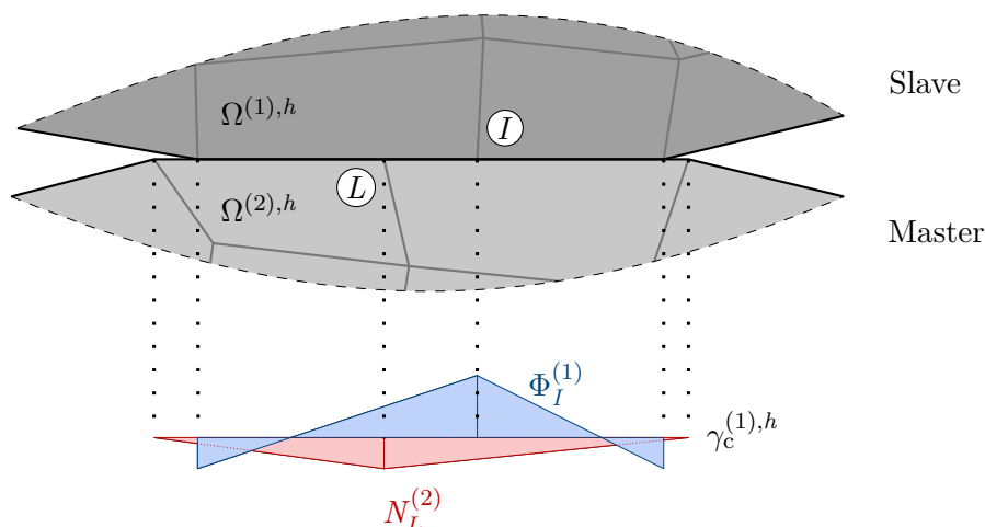
Abbildung 5.1: Ausschnitt eines diskretisierten Kontaktproblems mit Visualisierung der Formfunktionen der Knoten I und L .
