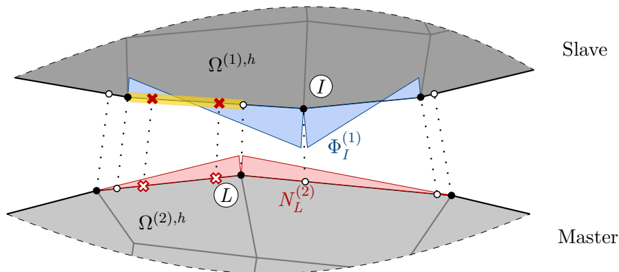
Abbildung 5.3: Veranschaulichung der Segmentierung und der segmentbasierten numerischen Integration für zweidimensionale Probleme. Darstellung der Integrationspunkte als Kreuze und der Kontakttrandknoten als Kreise. Tatsächliche Größen sind ausgefüllt dargestellt, projizierte Größen haben ein weiß ausgefülltes Symbol.
